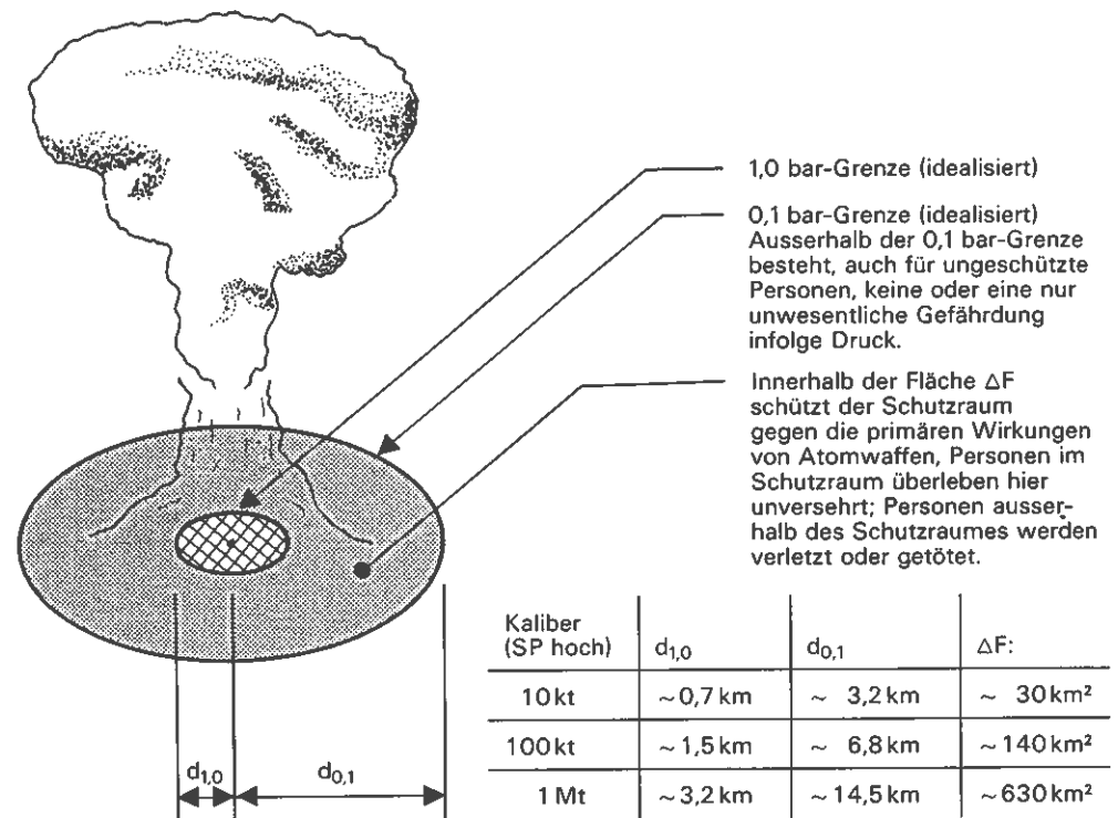
Figur 1.2-2 Idealisierte Wirkungsflehen des Überdrucks von 10 kt-, 100 kt-, 1 Mt-Atomwaffen bei optimalen Explosionshöhen
