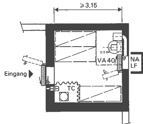
Figur 2.4-4 Grundrissform für 9 Schutzplätze (Bodenfläche \geq 10 \text{ m}^2 )
